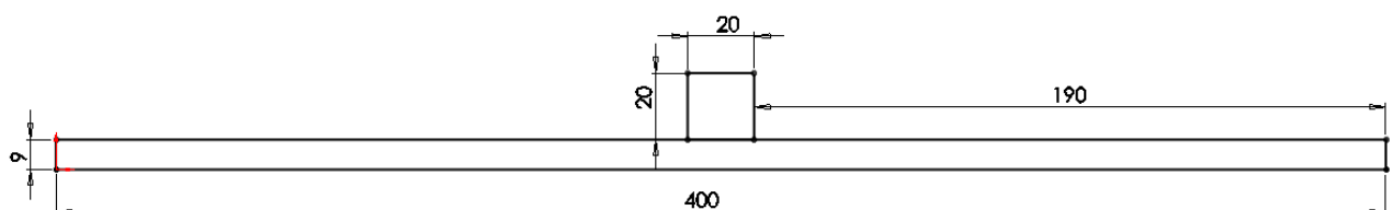
Figuur 2: geleide rail op de baan in aanzicht. maten in mm.
